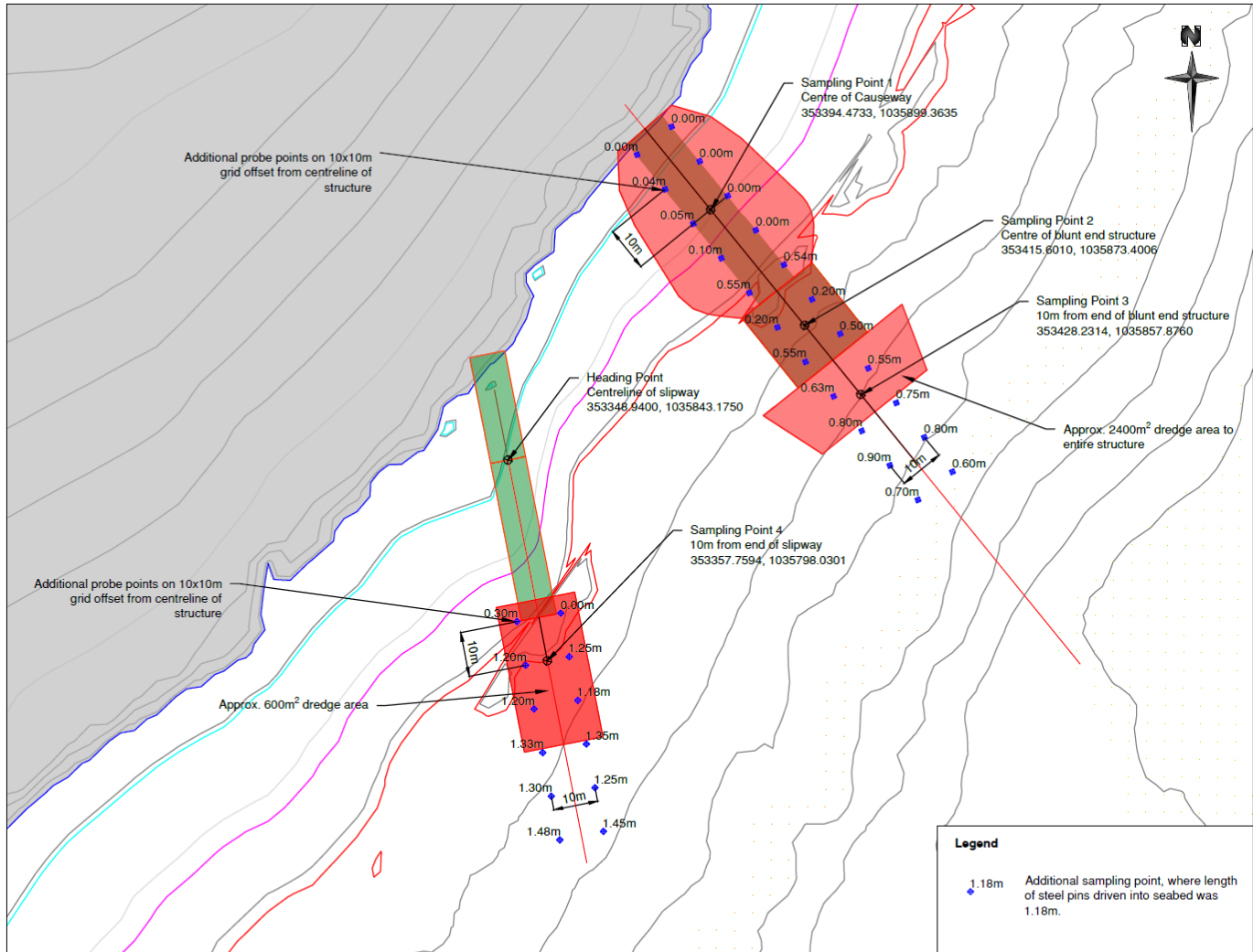
PLAN SCALE 1:1,000
